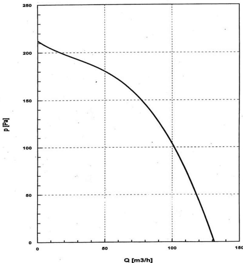
Tlaková charakteristika ventilátoru RATAS 3135
