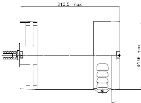
Ohne Lüfter
