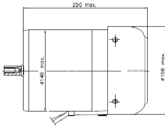
Mit Lüfter
